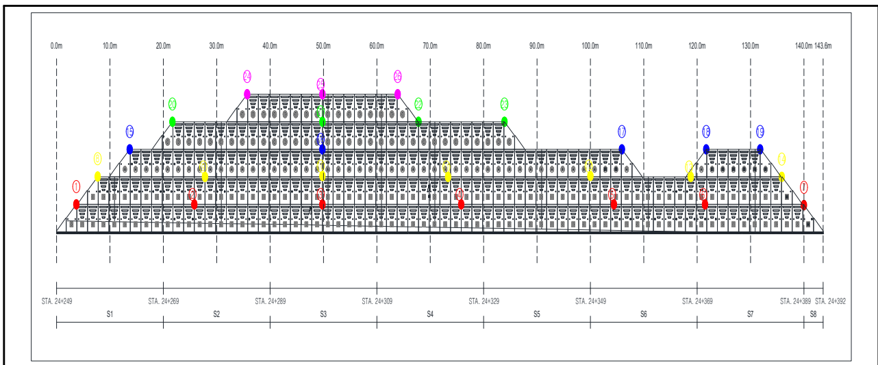
【그림 7.11】 측점분할 현황
