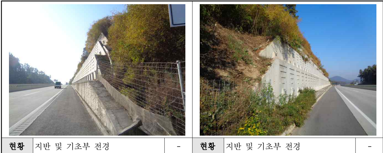
【사진 7.4】 지반 및 기초부 현황
